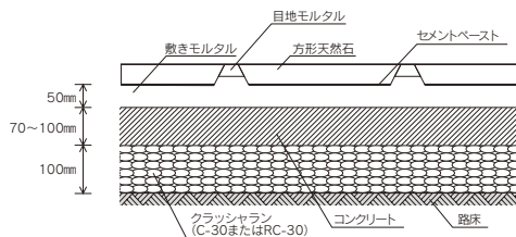
図2-1 ソレアド/アースウォーツ/桂林/ラジャスターン/カミニート/ジャワ鉄平/アクバル/ダナン/キュリオル/ラザリー/タフィー/オールドポルフィリー/ヴァリストーン参考施工図
