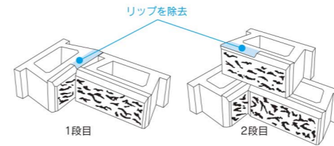
図 図-2-11 入隅コーナーの組積
