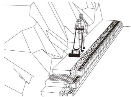
図 図-2-8 埋戻し土の締め固め
