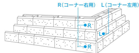
図 図-2-9 出隅コーナーの組積
