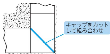
図 図-2-10 キャップの加工
