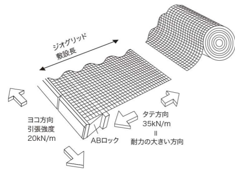
図 図-2-6 ジョグリッド敷設方向
