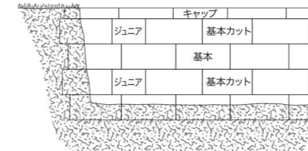
図 図-2-12 加工品の組積位置(正しい例)
