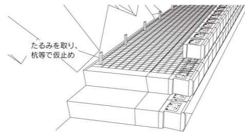
図 図-2-7 ジョグリッドの施工
