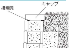
図 19-2-4 キャップ仕上げ
