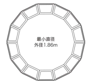
図 図-2-17 基本最小径
