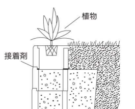
図 19-2-5 植栽仕上げ
