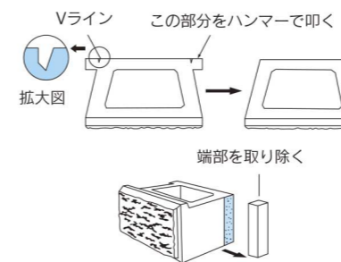
図 図-2-14 基本のカーブ用加工方法
