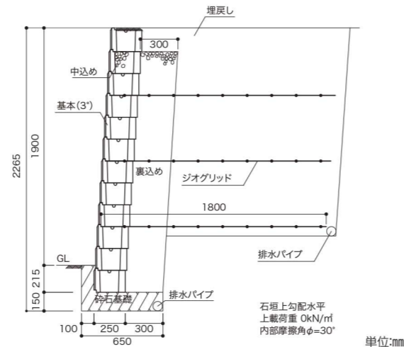
図 19-1-2 AB石垣の参考断面図
