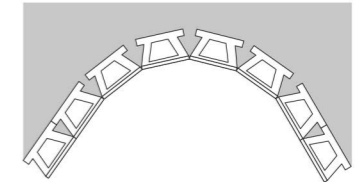
図 図-2-15 内曲がりカーブ
