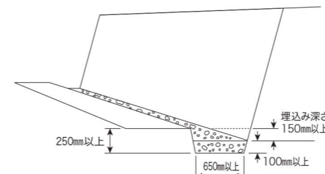
図 19-2-1 砕石基礎
