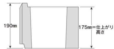
図 19-1-1 ABブロックの高さ
