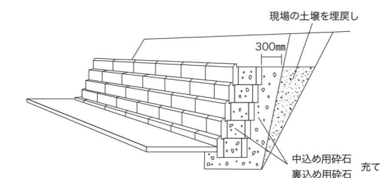
図 19-2-3 ABブロックの組積
