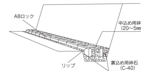
図 19-2-2 1段目の組積
