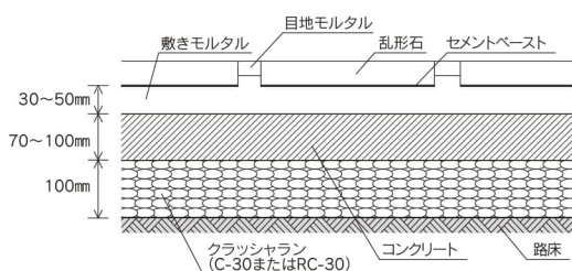
図1-1 乱形石参考施工図
