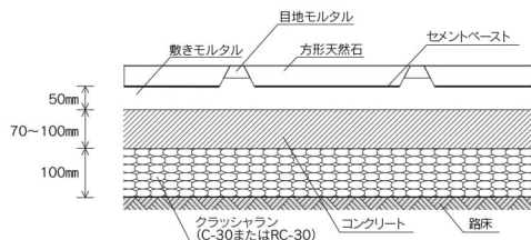
図2-1 ダナン/タフィー/ラザリー/アクバル/ヴァリストン/キュリオル/オールドポルフィリー/アースクォーツ/桂林/ラジャスターン/カミニート/ジャワ鉄平参考施工図
