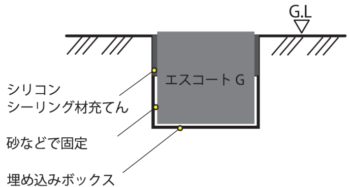
【参考断面図】
