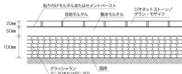
図4-1 ジオネットストーン／グラン・モザイク参考施工図
