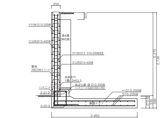
●RECOM 250※ 設計No.140/H=2,370mm
