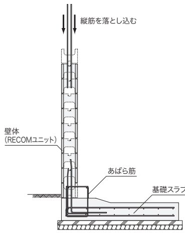
図 16-1-2 落とし込み配筋
