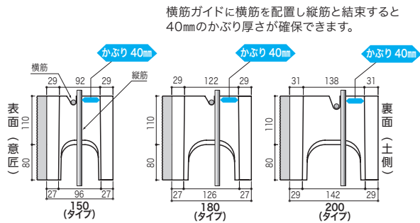
図 16-1-1 横筋ガイド
