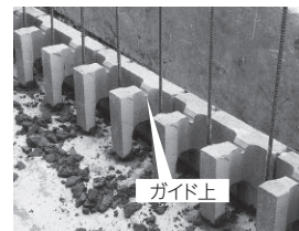
タイプE、L、Gの根付け
