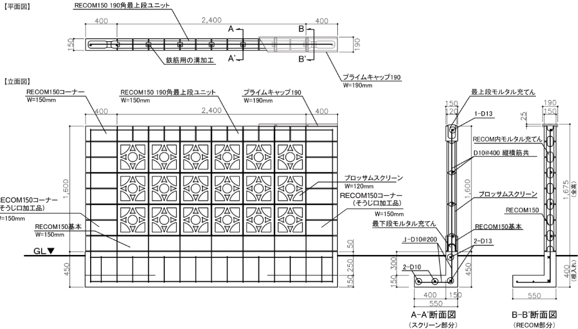
標準設計図(H=1,600mm)
