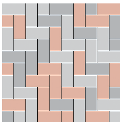
B-2 + G-2 + G-3 15個/㎡ + 25個/㎡ + 10個/㎡
