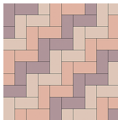
B-1 + B-2 + B-3 16.7個/㎡ + 16.7個/㎡ + 16.7個/㎡
