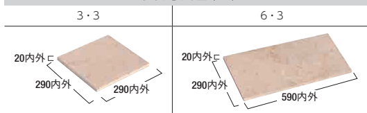
形状寸法図 (mm)
