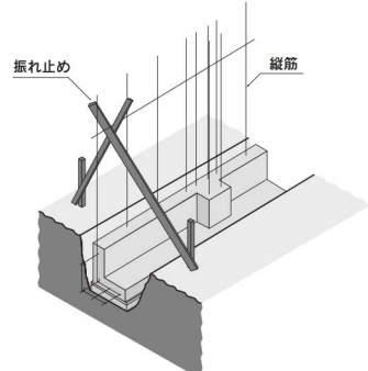
図③-2-6 L形の基礎+控柱用基礎
