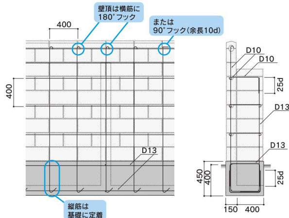
図③-2-9 ブロック塀の配筋例
