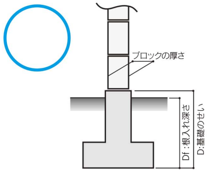
図③-2-3 正しい基礎
