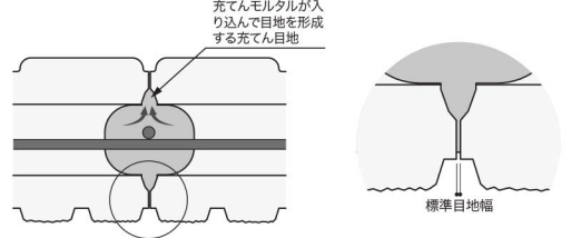
図3-2-13 充てん目地(化粧ブロック)
