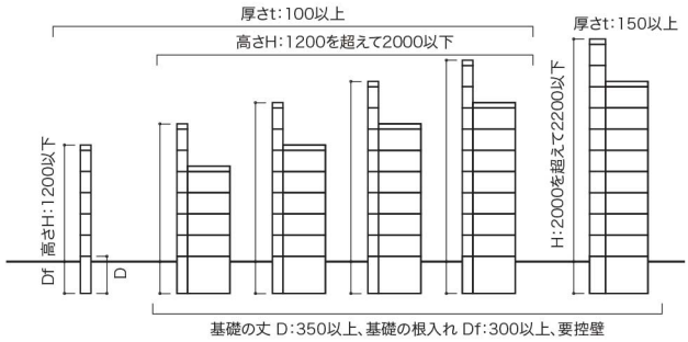
図2-1-1 建築基準法施行令による塀の例
