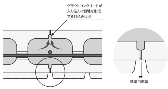
図3-2-12 打込み目地(型枠状ブロック)
