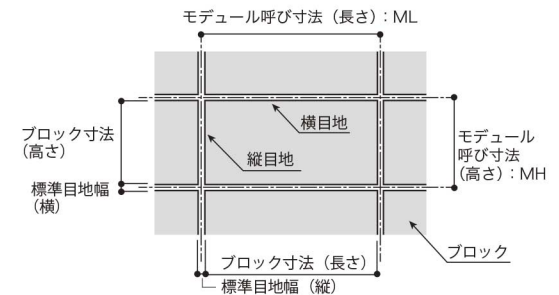
図：モジュール呼び寸法と標準目地幅
