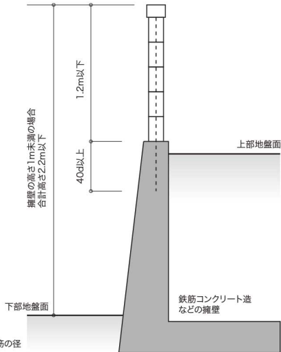
図2-2-8 擁壁の上の塀
