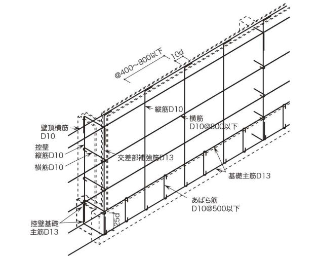
図2-2-2 配筋例
