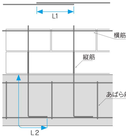
図3-1-3 重ね継手と定着長さの測り方
