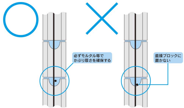
図③-2-8 かぶり厚さの確保
