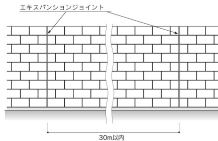
図2-2-10 エクspansionジョイントの設置
