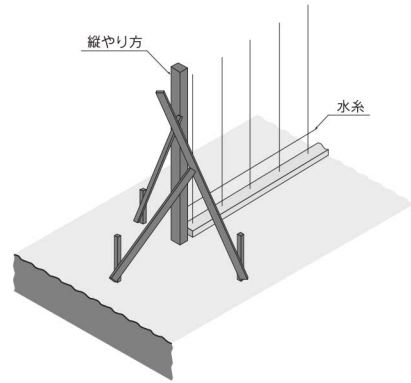
図③-2-7 縦やり方の例
