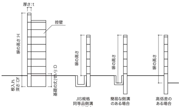
図2-1 塀の構成と高さ
