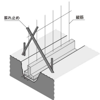
図③-2-4 逆T形の基礎
