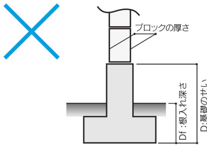
図③-2-2 根入れが不足している危険な基礎
