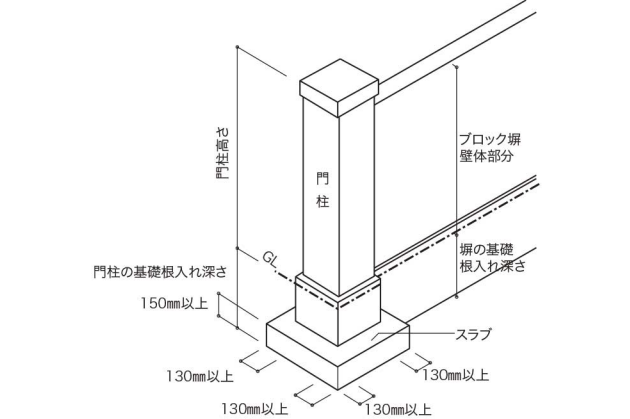
図2-2-3 門柱
