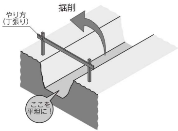
図3-2-1 掘削
