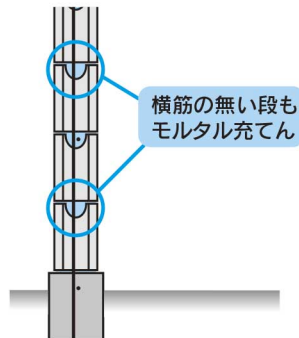
図③-2-10 基本形横筋のモルタル充てん
