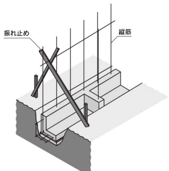
図③-2-5 L形の基礎
