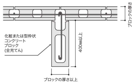
図2-2-5 控壁
