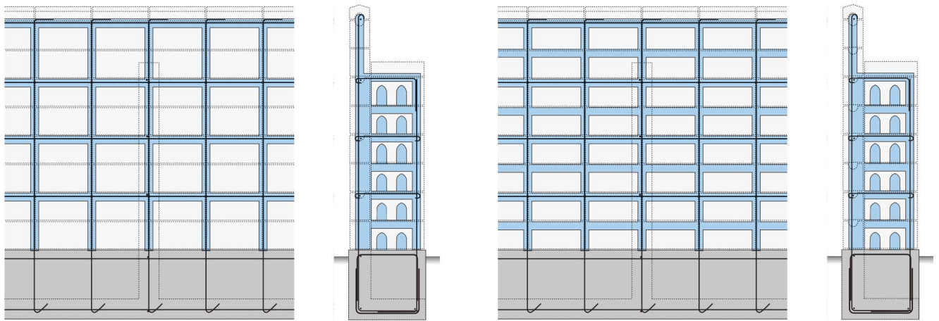
：モルタル充てん部 (基本&横筋:いも積みの場合)
