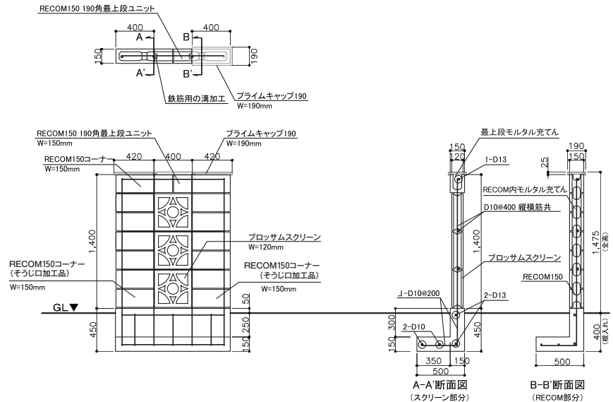
ブロッサムスクリーン H=1,400mm 組積構造図(一例) 単位:mm
