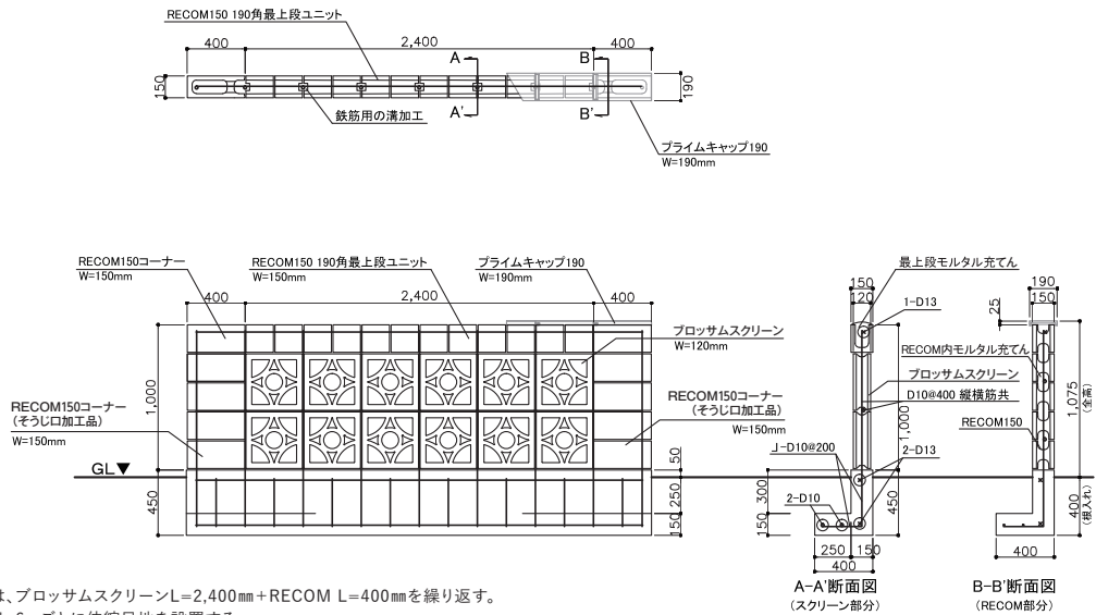
ブロッサムスクリーン H=1,000mm 組積構造図(一例) 単位:mm
