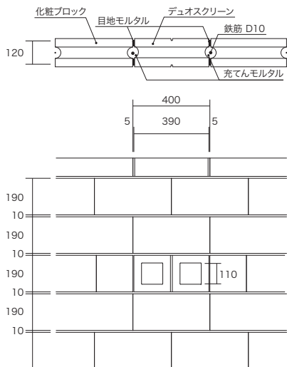
図3-1 デュオスクリーンの参考施工例
