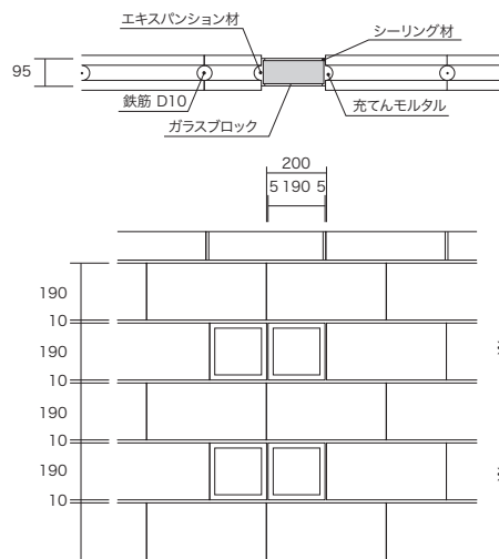
図3-2 ガラスブロックの参考施工例
