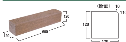
形状寸法図(mm)
