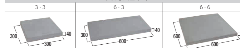
形状寸法図 (mm)
