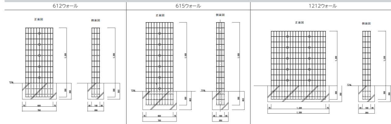
形状寸法図 (mm)
