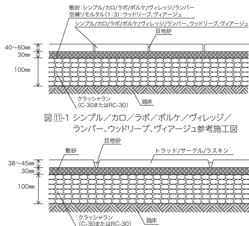
図 11-2 トラッド/サークル/ラスキン参考施工図
